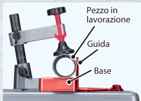
Supporto (opzionale)
